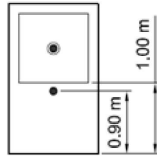
b) 具有较小玻璃面板的层门
